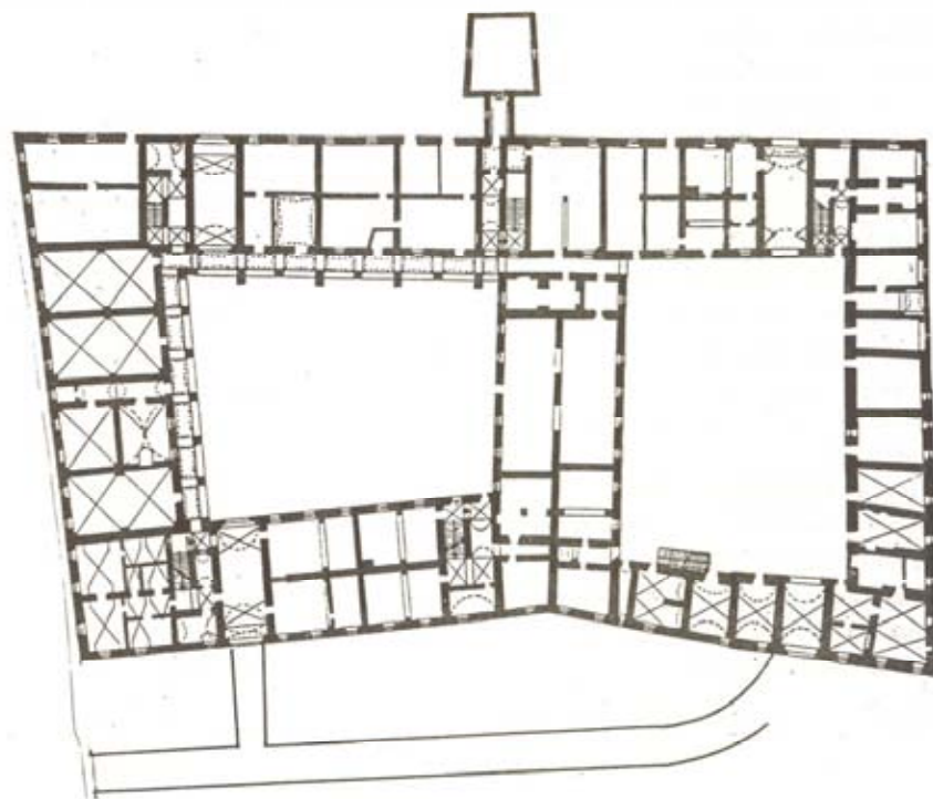
4. Az egykori kollégium épületének földszinti alaprajza. 1960-as évek.
