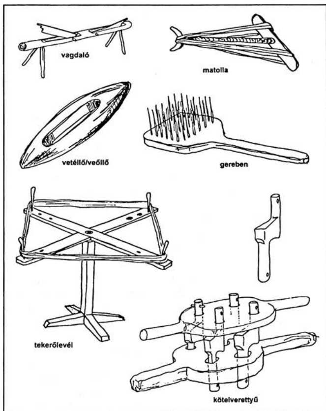
Kendermegmunkáló eszközök (Imecs László rajzai)
