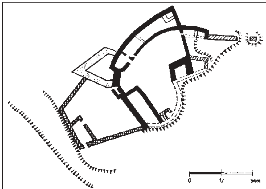
59. Tótfalud várának az alaprajza
