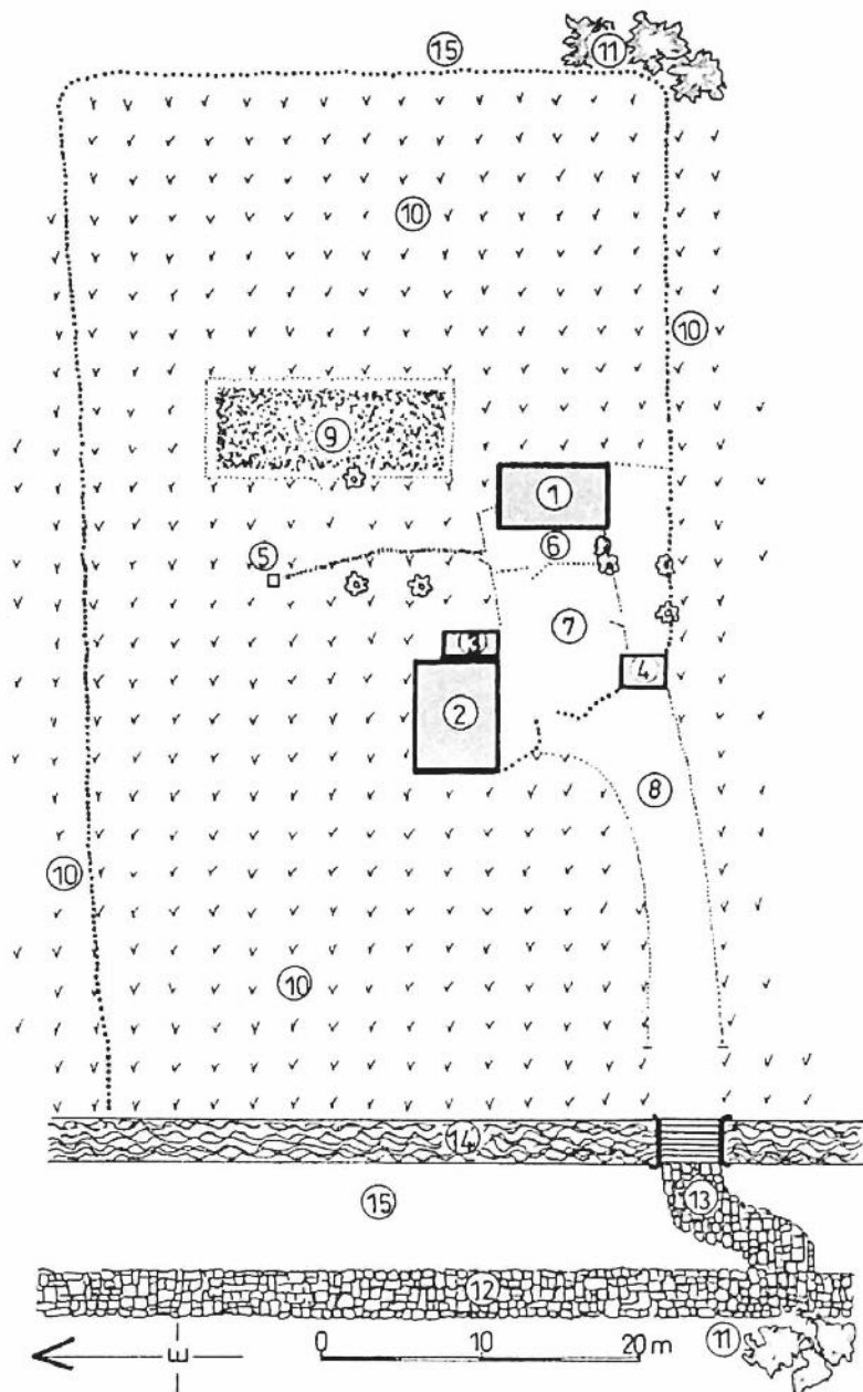
20. ábra. Baromudvaros elrendezései tanyai telephely a Varság patak völgyében. (4. sz. felmért telep). A számok jelentése: 1. ház, 2. csűr, 3. fákamra, 4. kicsi nyári ház, sütőház, 5. árnyékszék, 6. kicsi udvar, 7. nagy udvar, 8. bejáró ucca, 9. veteményes kert, szántó, 10. kaszáló, 11. erdő, 12. épített út, 13. épített lejáró, 14. Varság pataka, 15. meredek hegyoldal. A jelzett fák gyümölcsfák.
