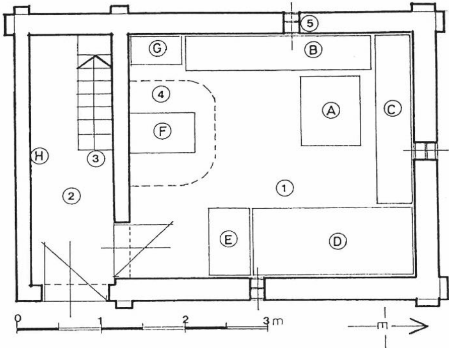
28. ábra. A 11. sz. felmért telephely oroszhegyi kicsi házának alaprajza a hajdani kuptor helyének jelölésével. A számok és betűk jelentése: 1. ház, 2. eresz, 3. létra, 4. köpadozat a hajdani kuptor helyén, 5. lyukablak, A. asztal, B. deszkapad, C. kanapé, fődeles padláda, D. ágy, E. szűszék , ácsolt láda, F. vastűzhely, G. fászláda, H. zakota , lim,lom.
